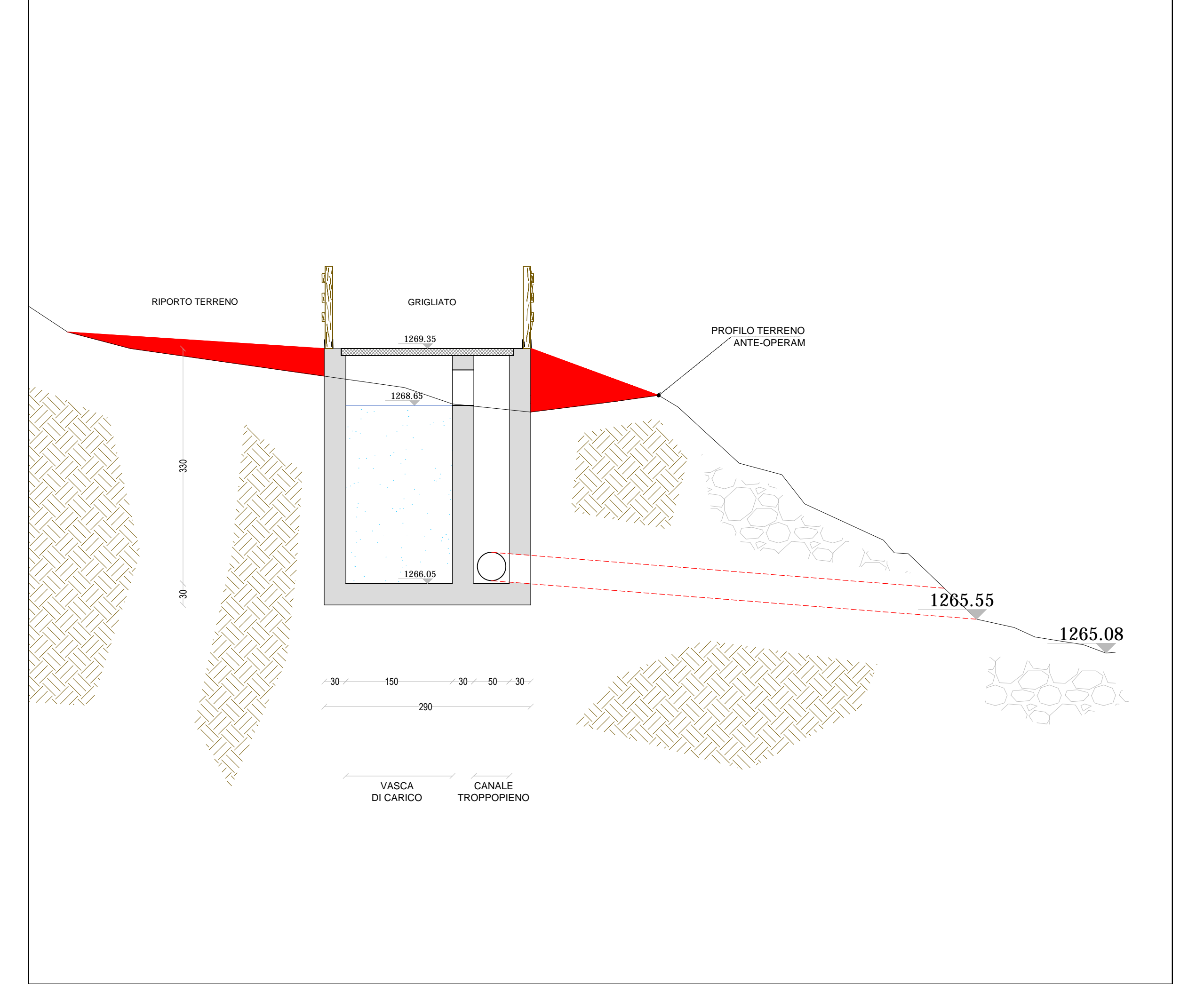
SEZIONE SCALA RISALITA ITTIOFAUNA - scala 1:50
