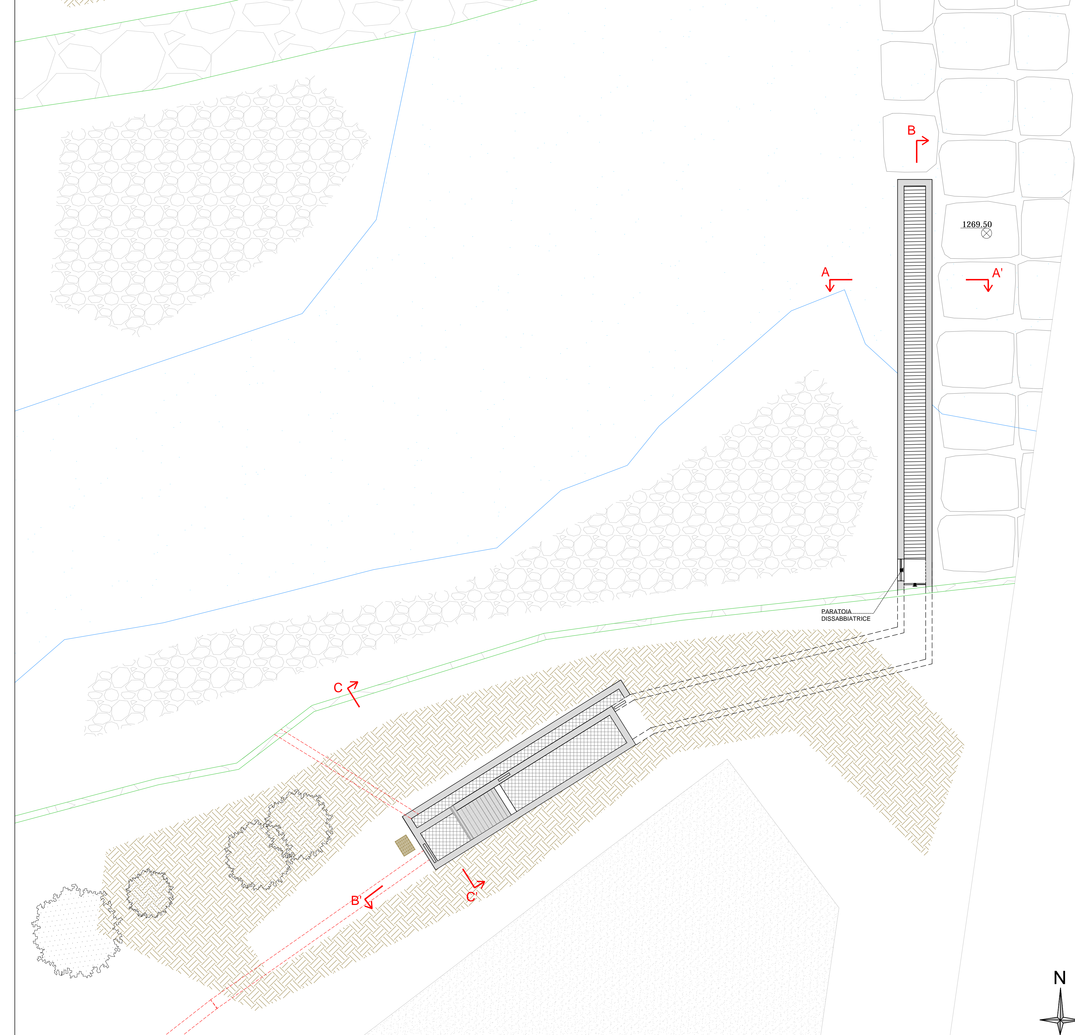
PLANIMETRIA OPERA DI PRESA A TRAPPOLA - scala 1:100
